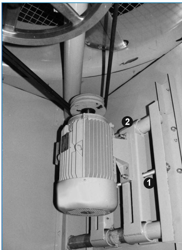
Verstellbare Motorkonsole
