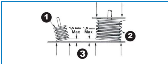
Riemenscheibenausrichtung Standardantriebe
