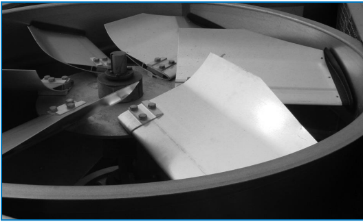
Ventilador axial
